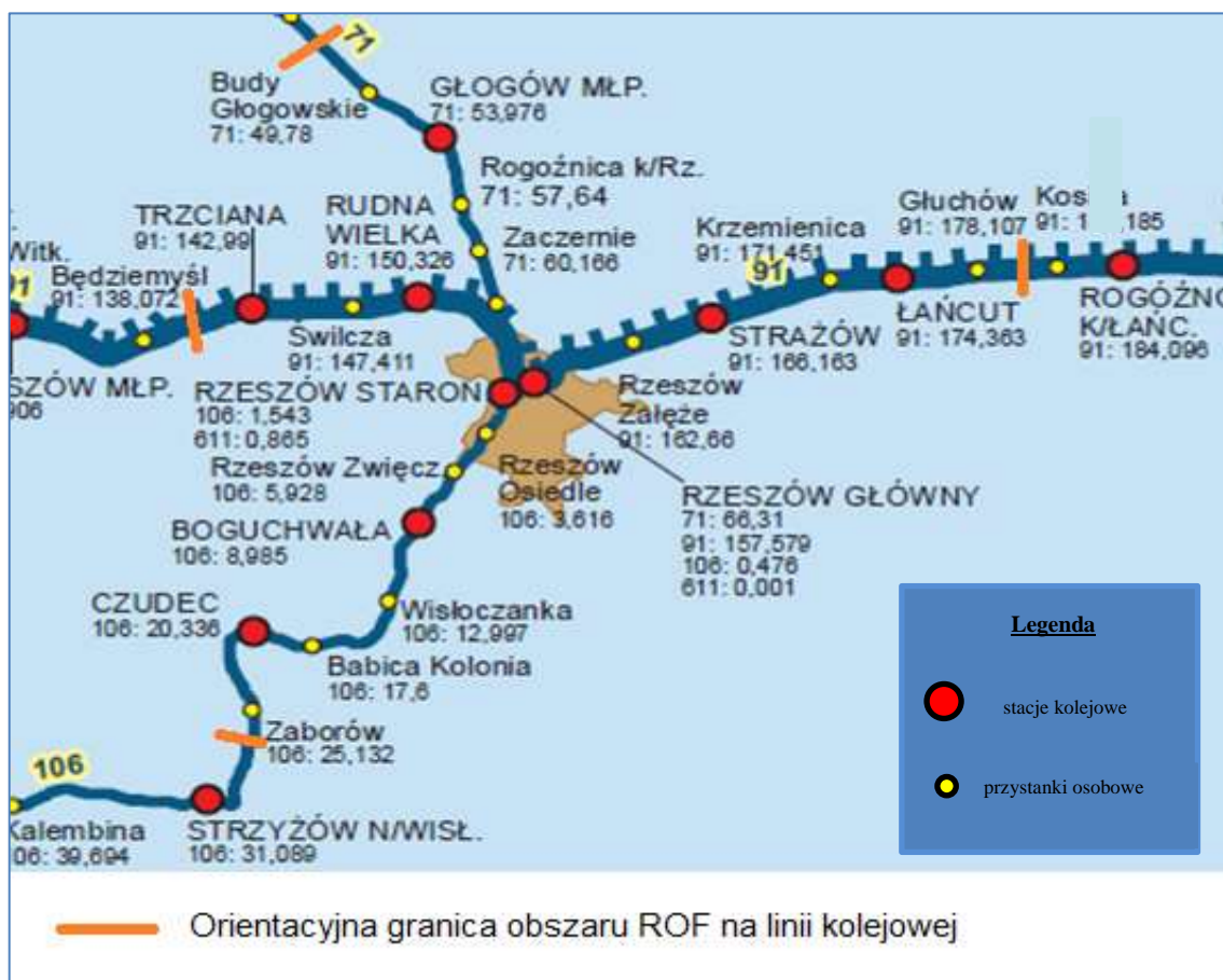
Rysunek 28. Układ sieci kolejowej przebiegającej przez teren ROF
